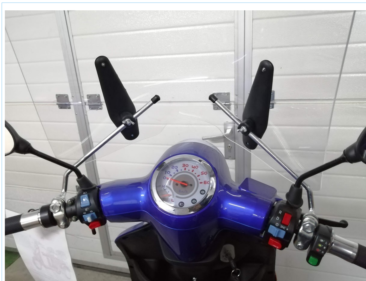
Imaginea 2: Exemplu de montaj pe o tricicleta electrica
