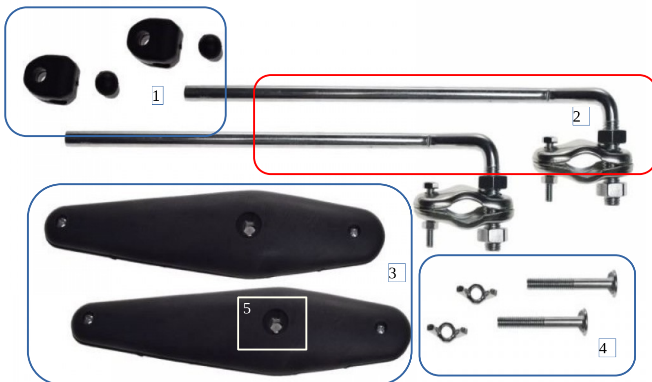
Imaginea 1: Piese componente
